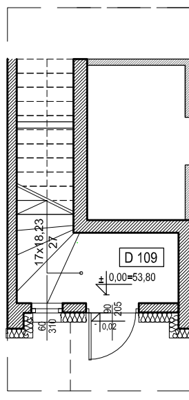
FRAGMENT RZUTU PARTERU Z WEJŚCIEM DO LOKALU 2
