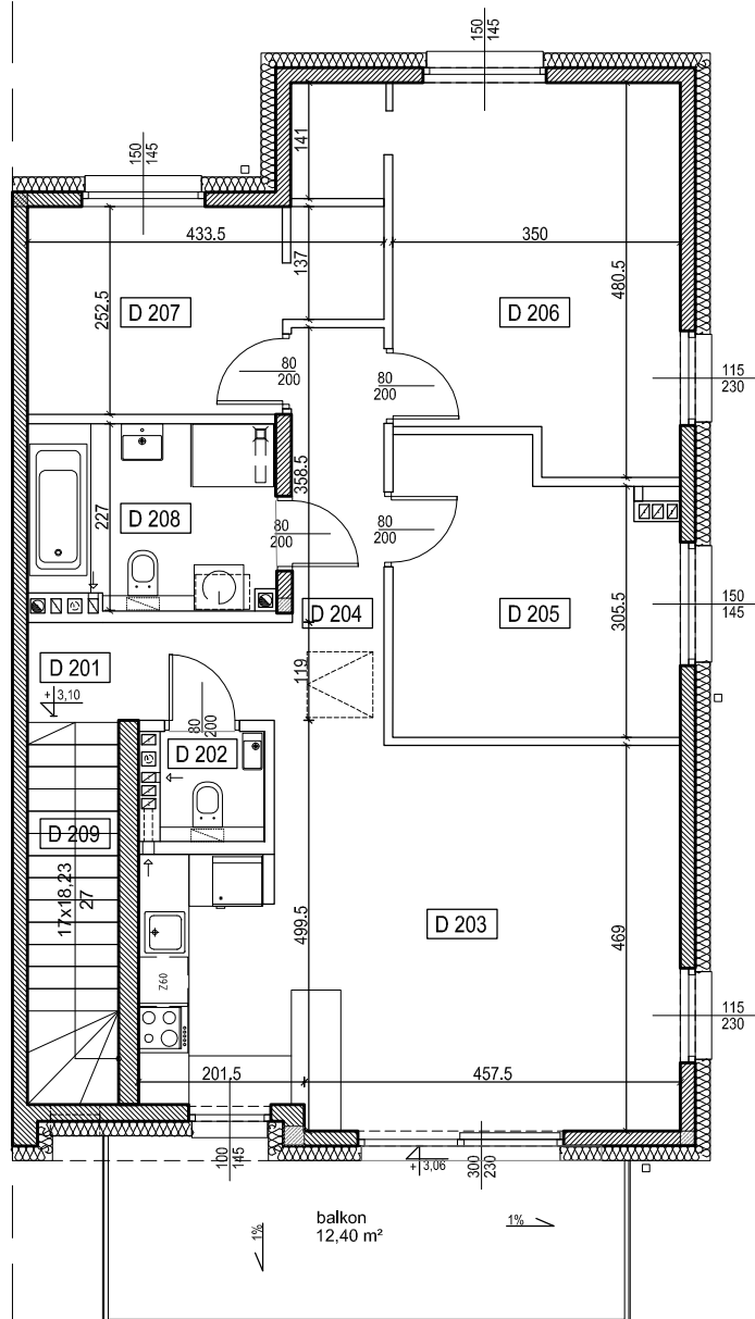
FRAGMENT RZUTU PARTERU Z WEJŚCIEM DO LOKALU 2
