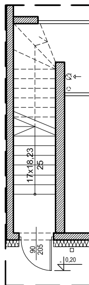
FRAGMENT RZUTU PARTERU Z WEJŚCIEM DO LOKALU "D"
